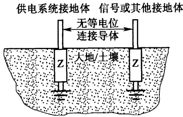
图 5 典型分开的接地
