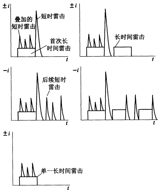
图 22 向上闪击可能的雷击组合
