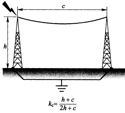
图 E.0.4 分流系数 k_c(3)
