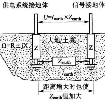
图 6 独立接地体与共用接地体之间的共模电位差
