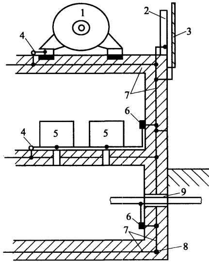
图 16 一钢筋混凝土建筑物内等电位连接的例子
