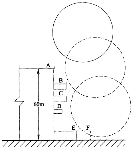
图 14 剖面示意
